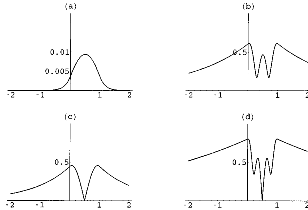
FIG. 2. (a) f_l^+(k_1, x) , (b) |f_l^+(k_2^+, x)| , (c) |f_l^+(k_3^+, x)| , and (d) |f_l^+(k_4^+, x)| .
