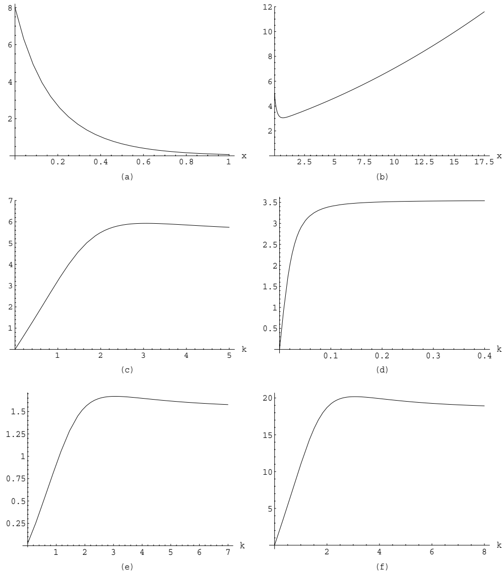
Figure 1. (a) Q(x) , (b) A(x) , (c) |P(k, l)| , (d) |Z(k, l)| , (e) |T(k, l)| and (f) |G(k, l; t)| of section 10.
